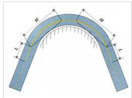
计算行车速度 V > 60\text{km/h} , L \geq 100\text{m} ; 计算行车速度 V \leq 60\text{km/h} , L \geq 50\text{m} 视距小于 M 值时, 双向车道道路在平曲线的中心线划法
