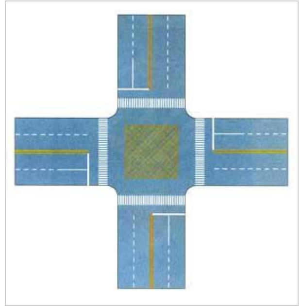
网状线
