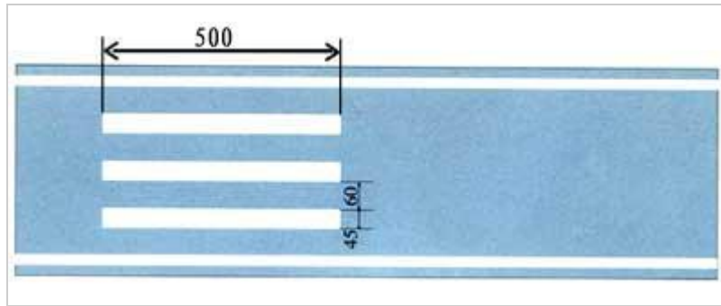
车距确认线尺寸
