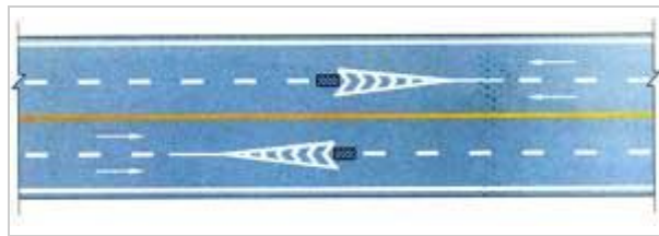
同方向二车道中间有障碍
