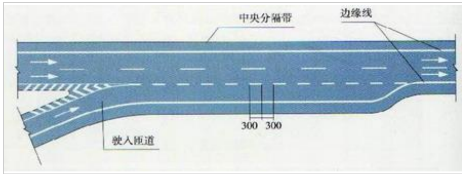
平行式入口标线
