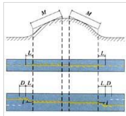
计算行车速度 V > 60\text{km/h} , L \geq 100\text{m} , D=40\text{m} , 斜率 i \geq 1:50 ;
