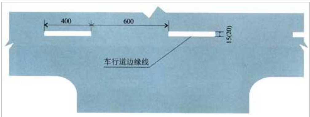
边缘线的尺寸 单位：cm
