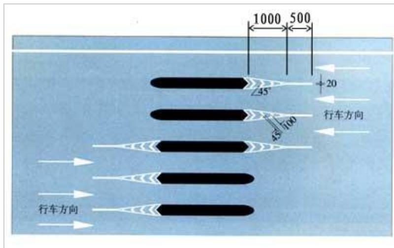
收费岛地面标线
