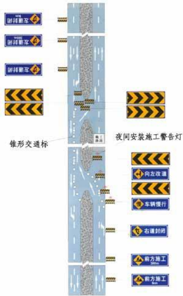
示例 7 高速公路一侧施工，利用中央分隔带紧急开口绕行时的设施布设例
