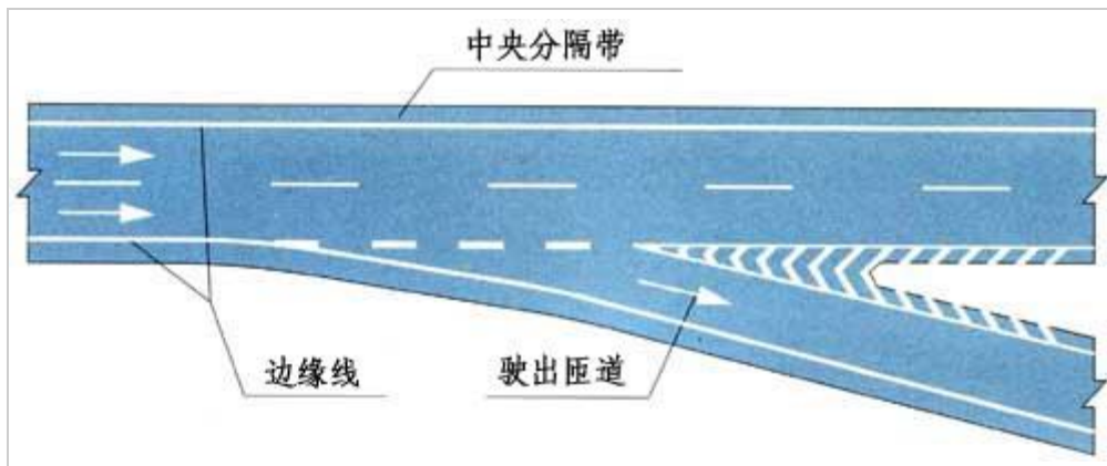
直接式出口标线
