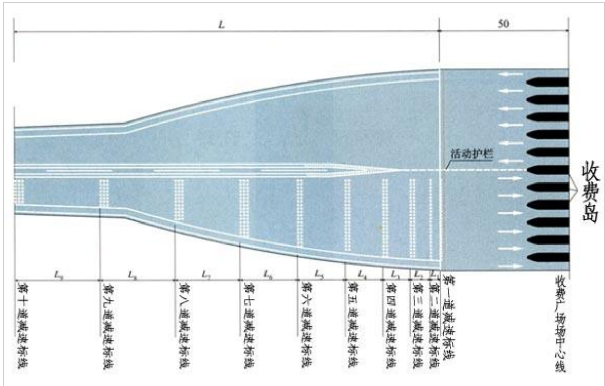
收费广场减速标线设置例
