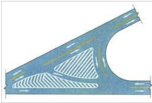
Y形路口导流线
