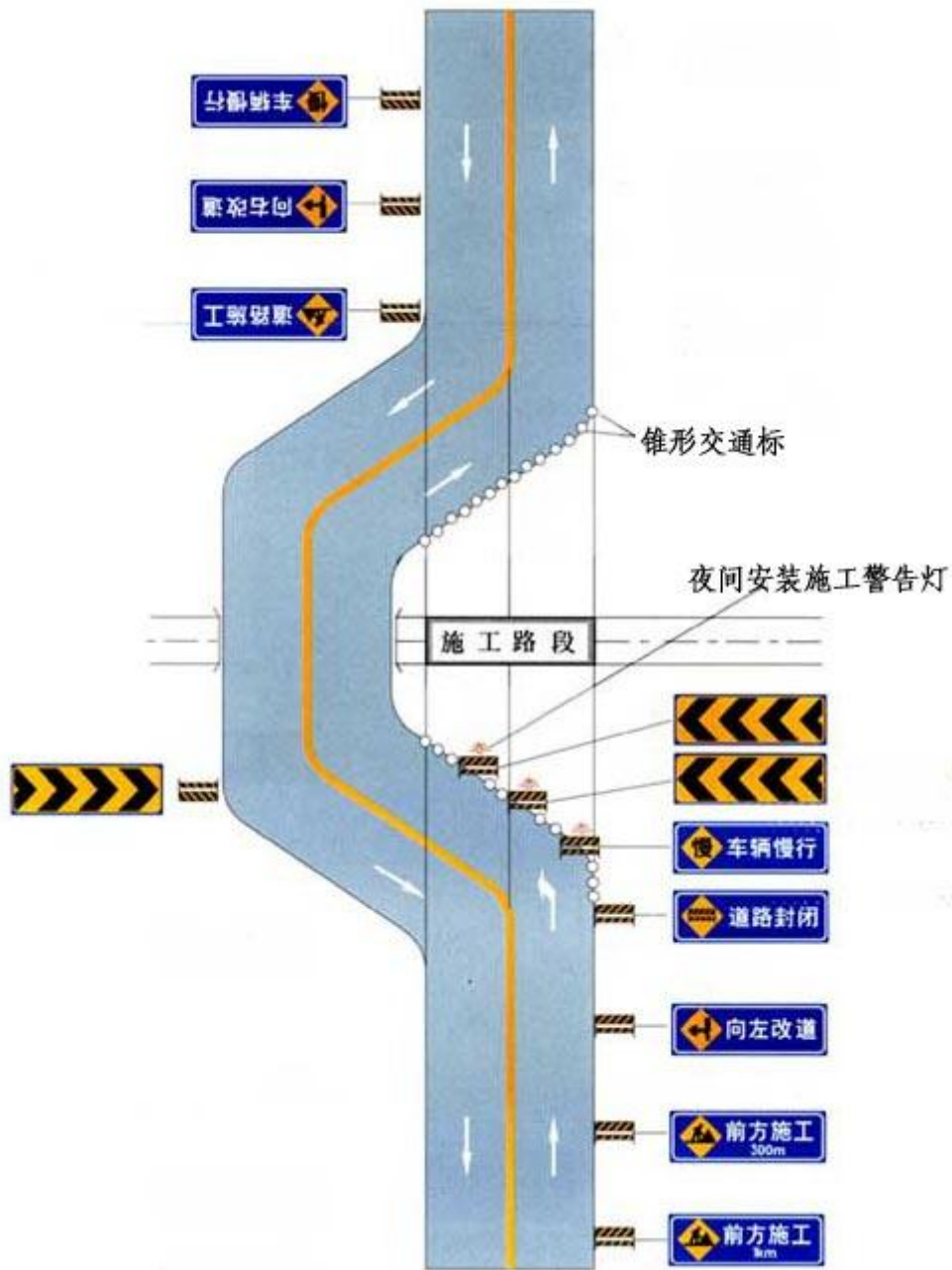
示例 3 改道施工时设施布设例
