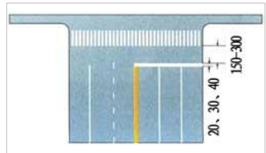
停止线的尺寸 单位:cm
