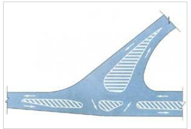
斜交丁字路口导流线
