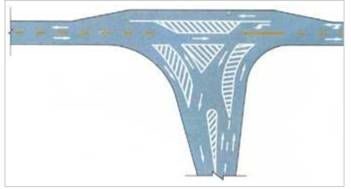
复杂行驶条件丁字路口导流线
