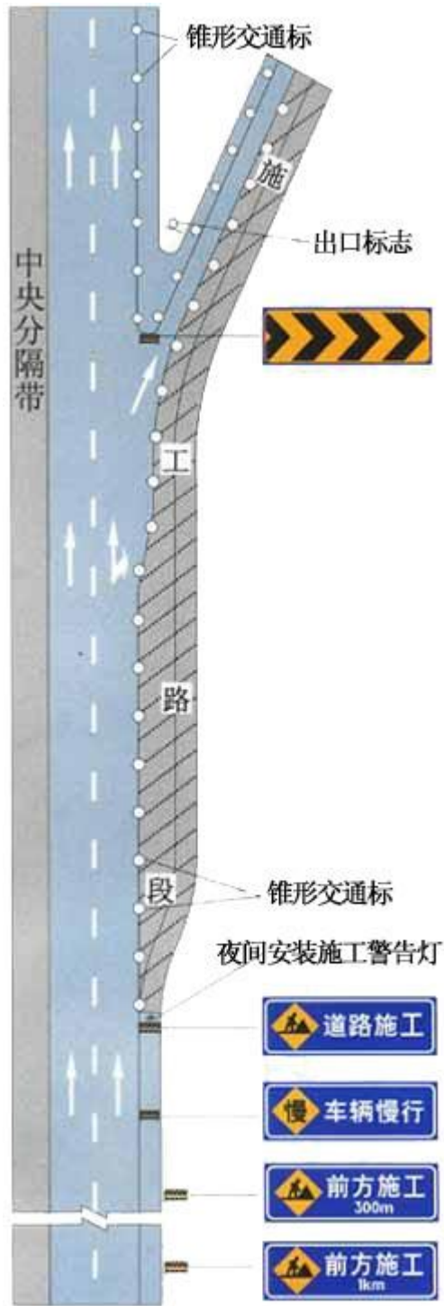
示例 13 高速公路出口减速车道施工时的设施布设例
