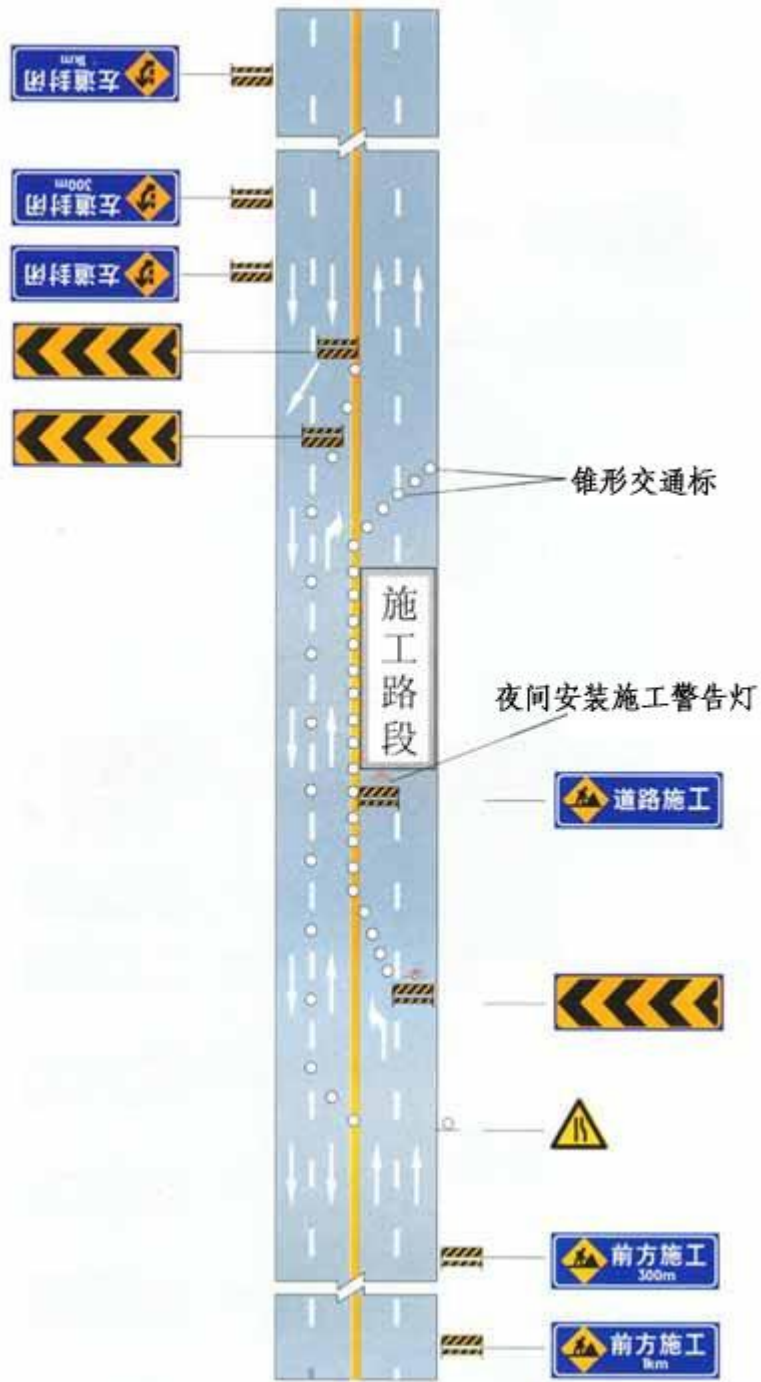
示例 4 四车道以上道路一侧路面施工时设施布设例
