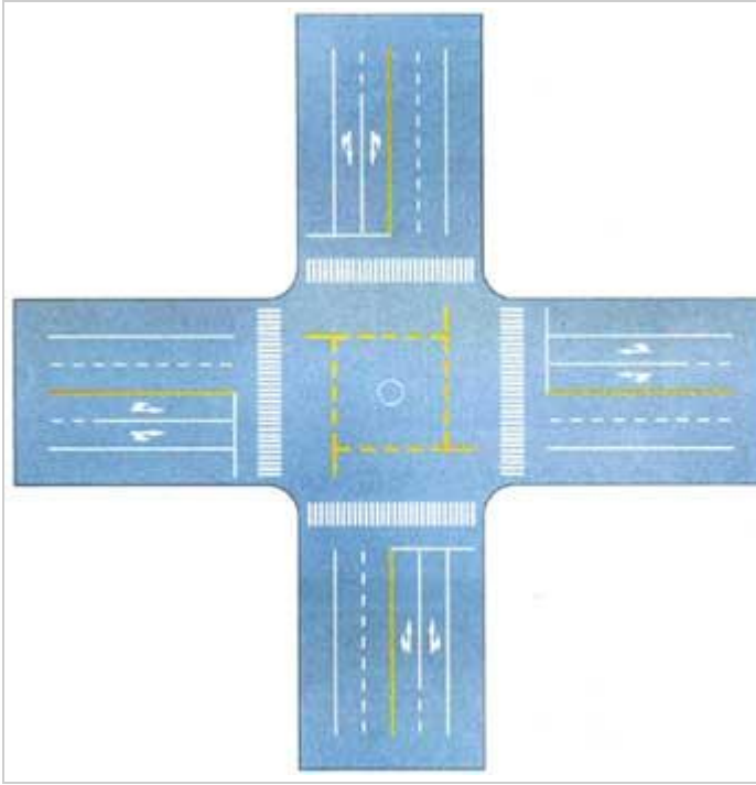
非机动车禁驶区标线
