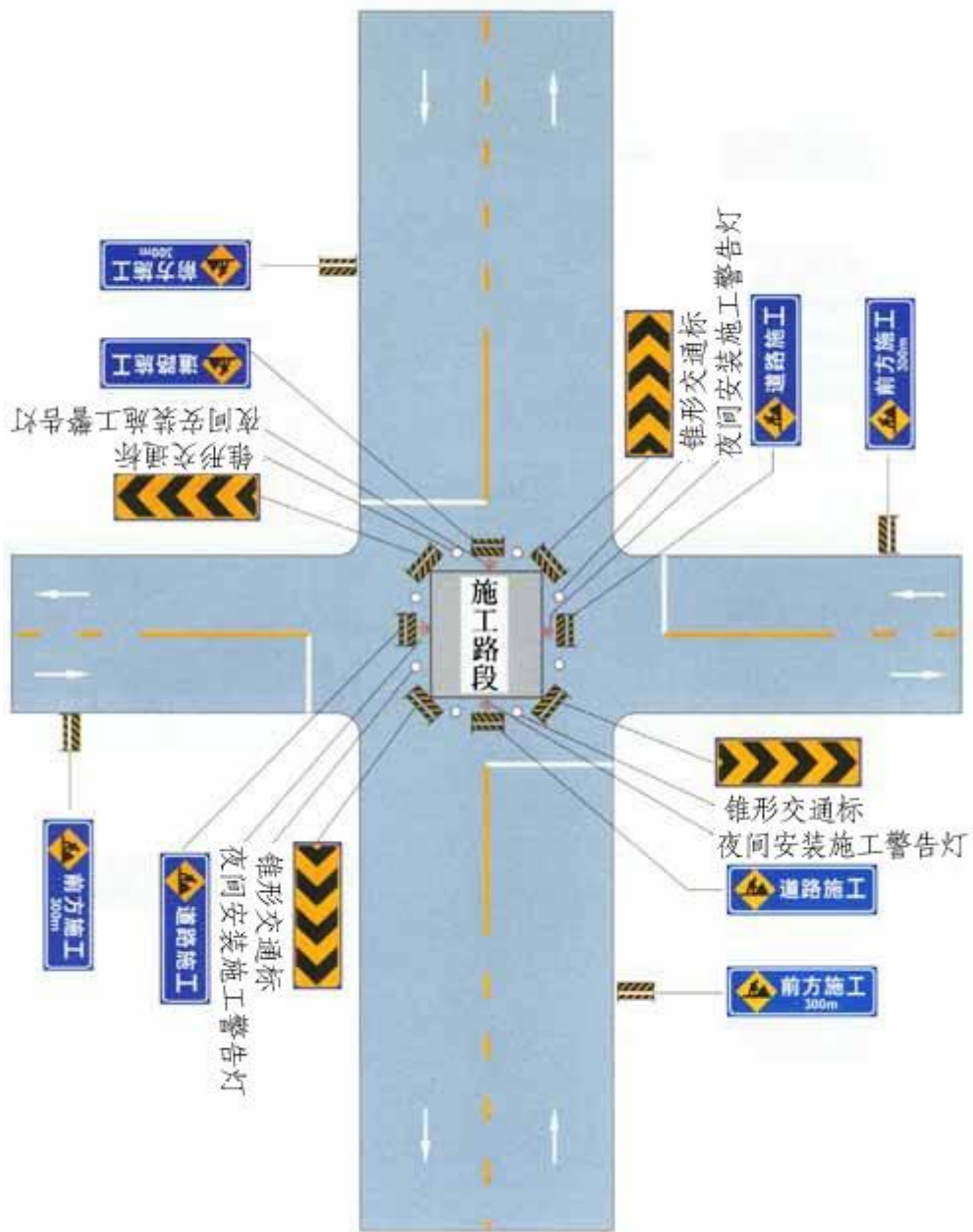
示例 10 市区道路交叉口中心线附近施工时的设施布设例
