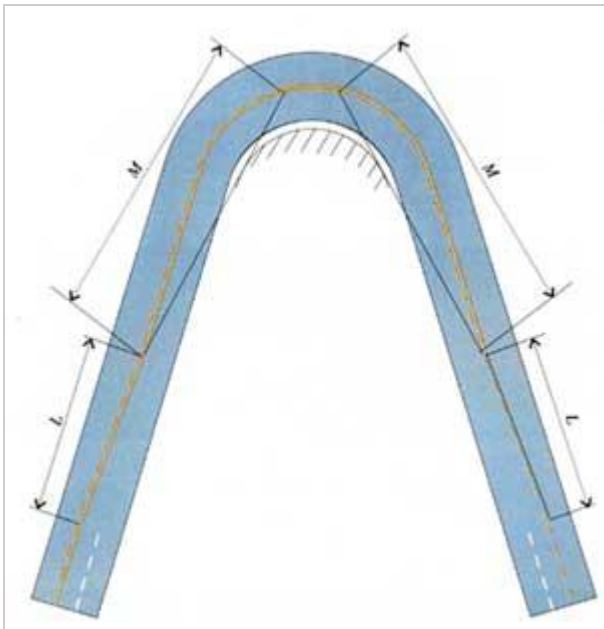
计算行车速度 V > 60\text{km/h} , 斜率 i \geq 1:50 ; 计算行车速度 V \leq 60\text{km/h} , 斜率 i \geq 1:20 ; M =最小视距
