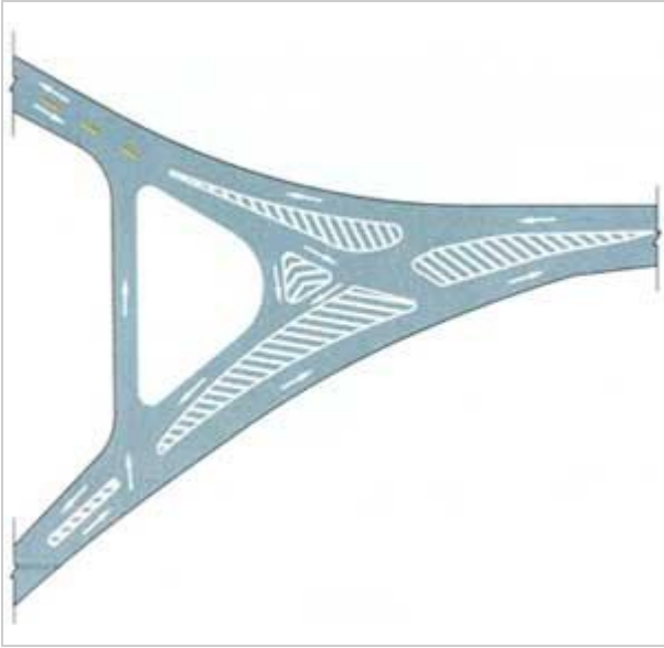
不规则路口导流线
