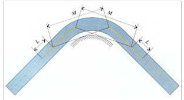
计算行车速度 V > 60\text{km/h} , L \geq 100\text{m} ; 计算机车速度 V \leq 60\text{km/h} , L \geq 50\text{m} 视距小于 M 值时, 双向两车道道路在平曲线的中心线划法
