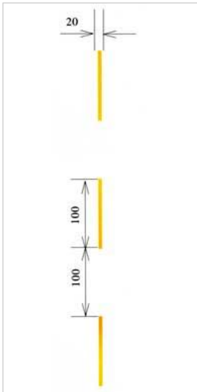
禁驶区标线尺寸 单位:cm
