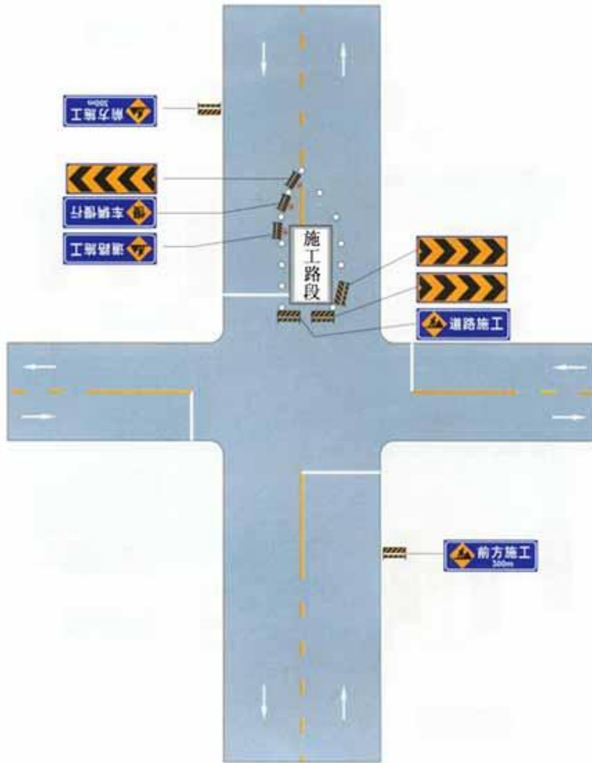
示例 9 市区道路交叉口中心线附近施工时的设施布设例
